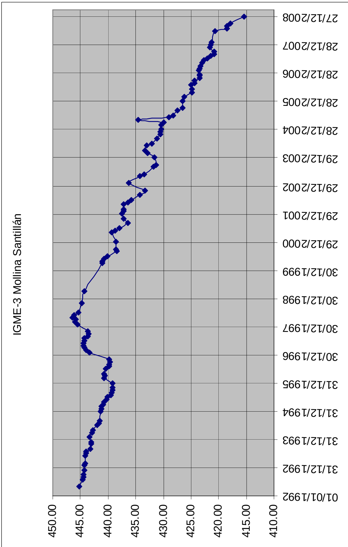
Figura 2.a. Hidrograma del sondeo de observación piezométrica 1642-3-109 -IGME 3 Molina Santillán-
